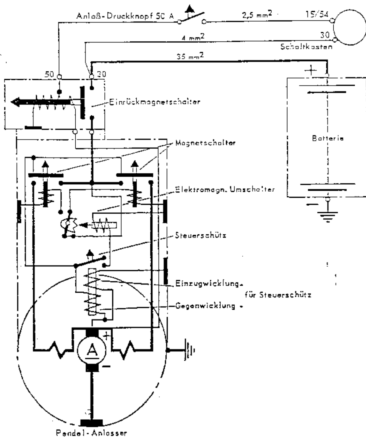
Schaltung des BOSCH-Pendelanlassers für elektromagnetische Einrückung
