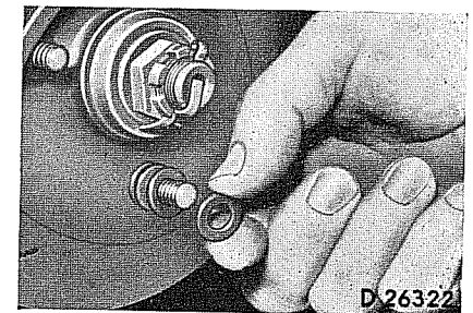
Einstellscheiben für Windflügelriemen
