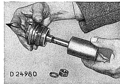
Schmierölfilter zerlegen
