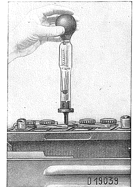
Prüfen der Säuredichte und des Ladezustandes der Batterie
