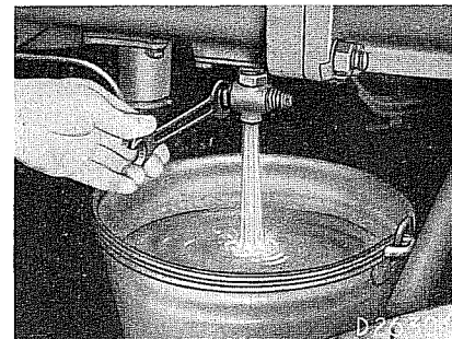
Kühlwasser ablassen
