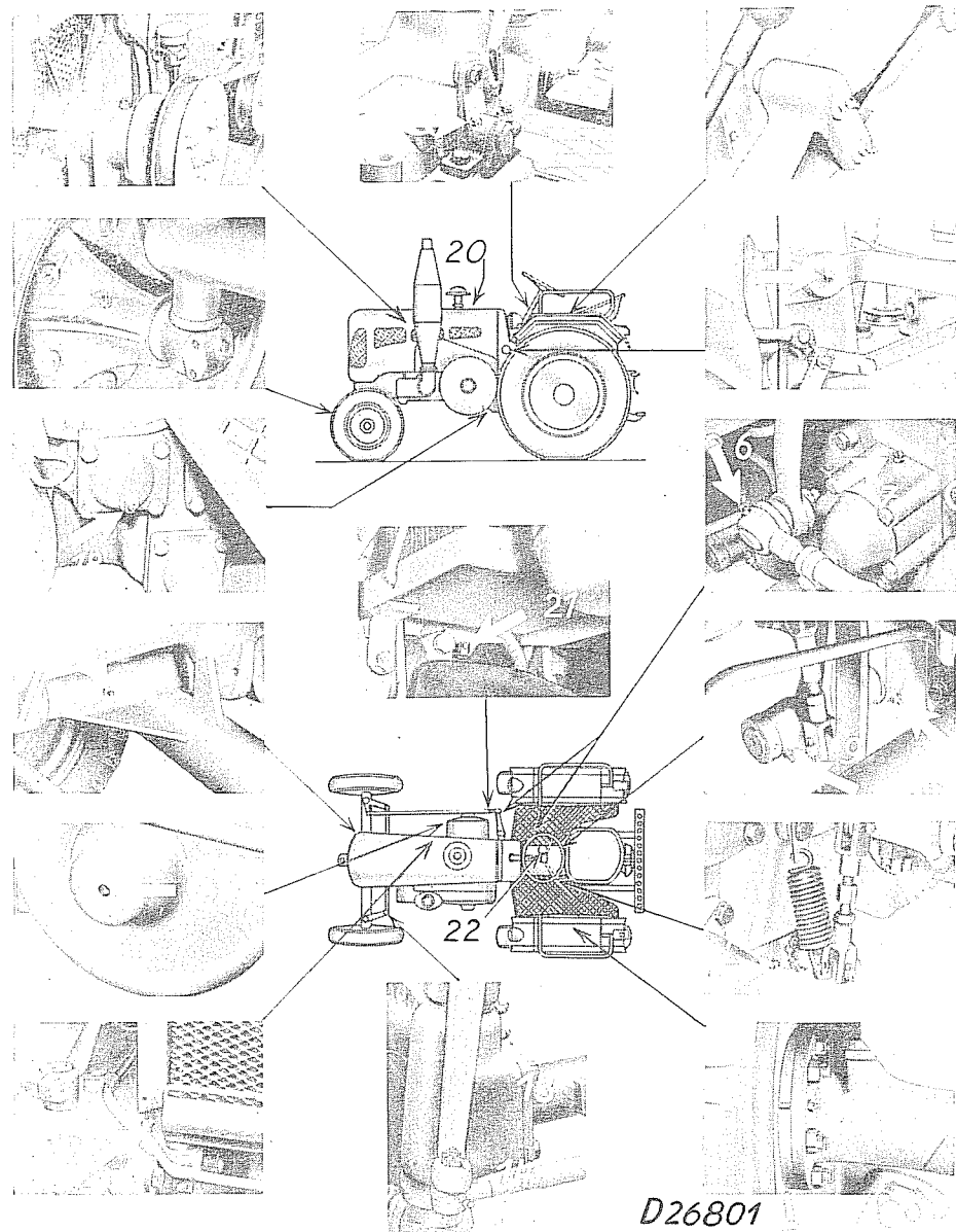
Schmierstellen des Bulldog
