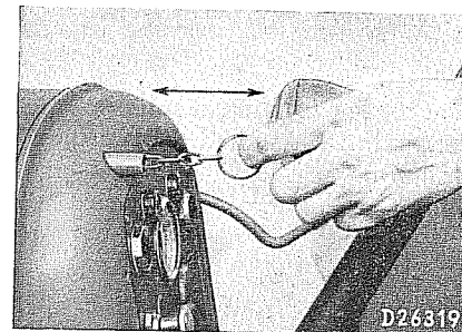
Kühlerrollo — Betätigung
