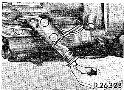
Ausbau des Ölfilters im Kurbelgehäuse
