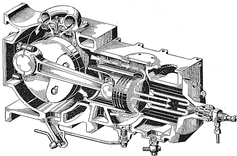
Motor, Schnitt
