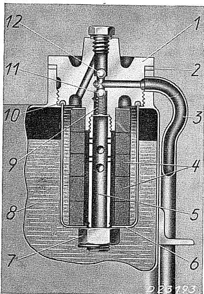
Schmierölfilter, Schnitt
