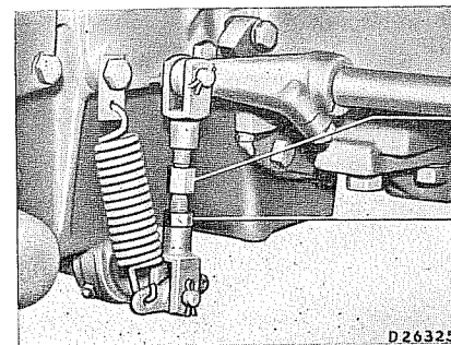
Nachstellschraube
