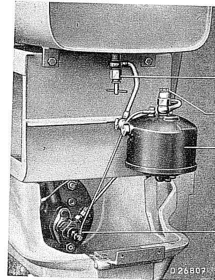
Kraftstoff-Absperrventil
