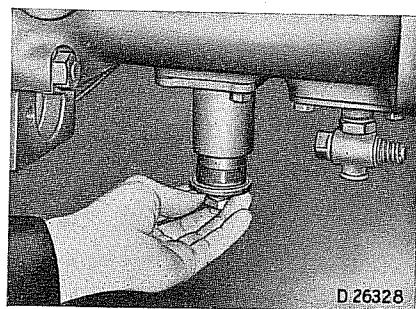
Zylindereinsatz herausnehmen
