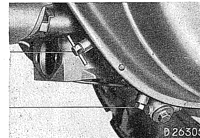
Kontroll- und Ablafschrauben für Pumpenantrieb
