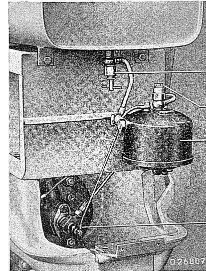
Kraftstoff-Absperrventil
