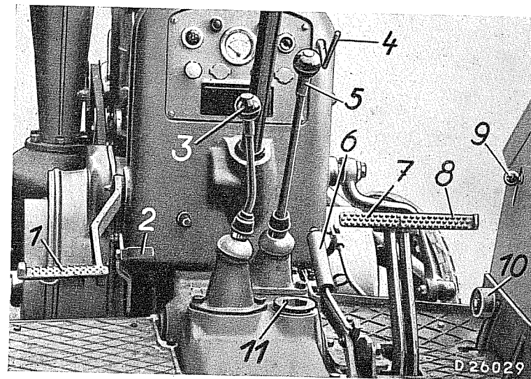
Fahrerstand
