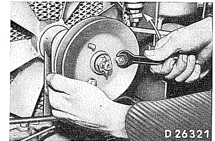
Riemenrollenhälfte abschrauben
