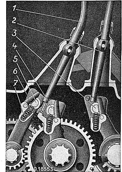
Gangschaltung, Schnitt
