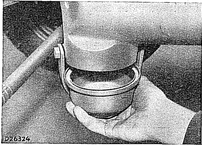
Auspuff-Sammeltopf abnehmen
