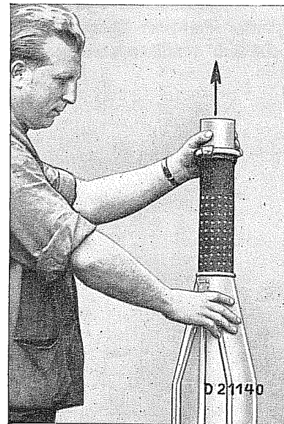
Ausziehen des Funkenschutzsiebes
