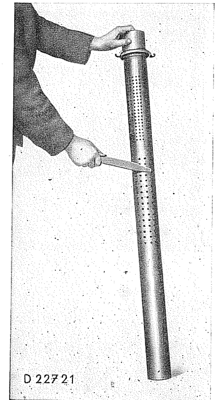
Reinigen des Funkenschutzsiebes
