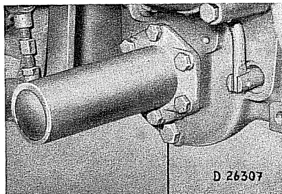
Getriebeöl-Ablafschraube
