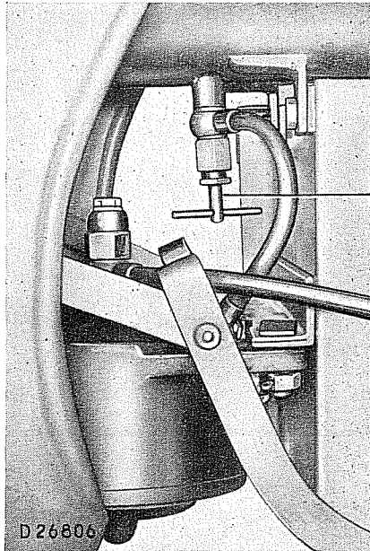
Kraftstoff- absperrentil
